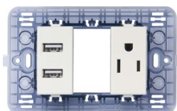
BM0236 2.1A/5V 15A/125V
